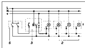
3. Aansluiting via serieschakelaar voor permanente verlichting en automatische werking
